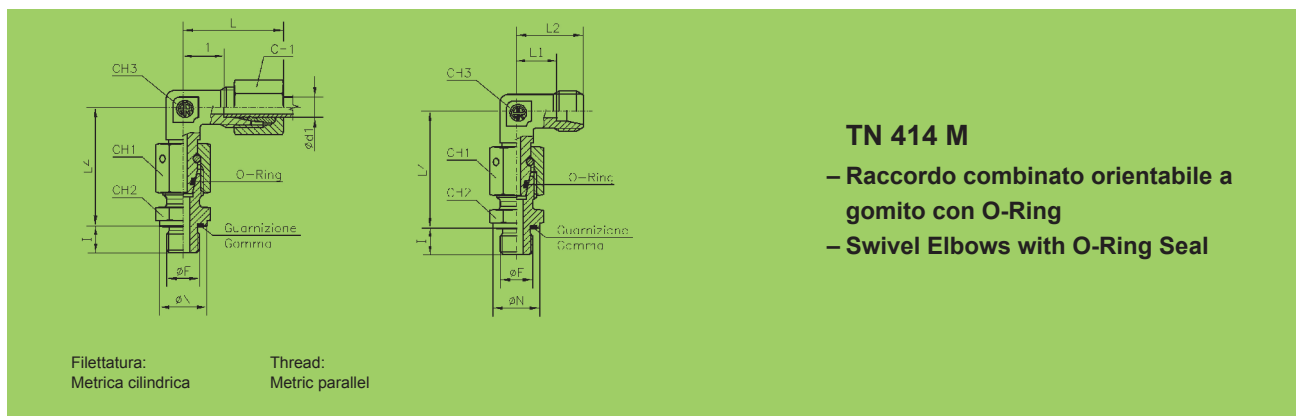
Forma E DIN 3852 Foglio 11
