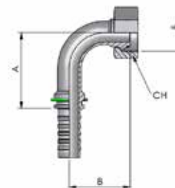
DRY-SPIRAL METRIC FITTINGS 24° INSERTI METRICI 24° DRY-SPIRAL
