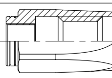
2000-04 ОБЖИМНАЯ ВТУЛКА R2 AT Рукав без снятия оболочки
