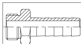
5074 РУКАВНАЯ МУФТА, BSP M ЛАТУНЬ
