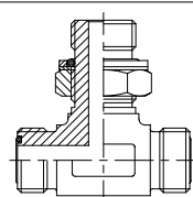
7741 РЕГУЛИРУЕМЫЙ Т- ОБРАЗНЫЙ ФИТИНГ ORFS X ORFS X НАРУЖНАЯ РЕЗЬБА G (BSP) с кольцевым уплотнением и шайбой
