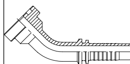
4258 Фитинг 45°, фланцевый, SAE J518 Код 62
