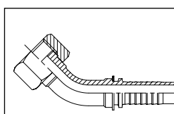
4292~2 Фитинг угловой 45°, унифицированная внутренняя резьба, уплотнение ORFS Накидная гайка
