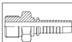
4215 Фитинг SAE-O, унифицированная наружная резьба, с уплотнительным кольцом
