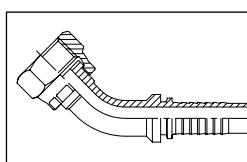
4292 Фитинг угловой 45°, унифицированная внутренняя резьба, уплотнение ORFS Обжимная гайка
