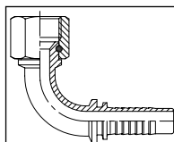
4216~1 Фитинг JIC, унифицированная внутренняя резьба, угловой 90°, коническое уплотнение 74° Гайка с упорной проволокой
