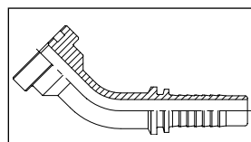
4248 Фитинг 45°, фланцевый, SAE J518 Код 61
