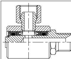
5594 ПОВОРОТНЫЕ МУФТЫ ВЫСОКОГО ДАВЛЕНИЯ, 90°
