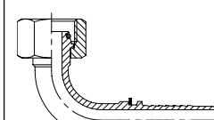
4274~2 Фитинг поворотный, угловой 90°, внутренняя М-резьба, коническое уплотнение 24°, с уплотнительным кольцом, Накидная гайка
