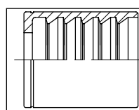
4200-03 ОБЖИМНАЯ ВТУЛКА EN1SN, 2SC БЕЗ СКОСА ЗУБЬЕВ
