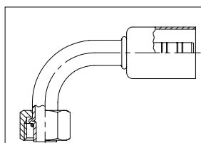
5703 UN 90° FS с уплотнительным кольцом Для рукава AC 1445
