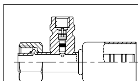
5702 UN FS с уплотнительным кольцом/клапанами Для рукава AC 1445
