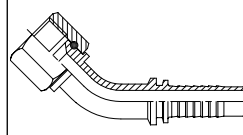
4217~1 Фитинг JIC, унифицированная внутренняя резьба, угловой 45°, коническое уплотнение 74° Гайка с упорной проволокой
