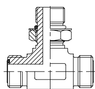
7742 РЕГУЛИРУЕМЫЙ Т-ОБРАЗНЫЙ ФИТИНГ ORFS X ORFS X НАРУЖНАЯ РЕЗЬБА UNF, С СОЕДИНЕНИЕМ SAE O с кольцевым уплотнением и шайбой
