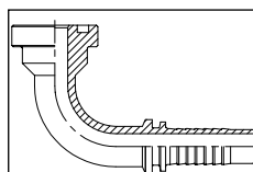
4254 Фитинг 90°, фланцевый, SAE J518 Код 62
