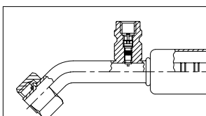
5706 UN 45° FS с уплотнительным кольцом/клапанами Для рукава AC 1445
