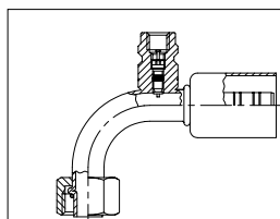
5704 UN 90° FS с уплотнительным кольцом/клапанами Для рукава AC 1445
