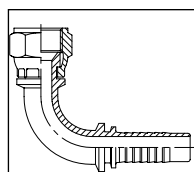
4216 Фитинг JIC, унифицированная внутренняя резьба, угловой 90°, коническое уплотнение 74° Обжимная гайка
