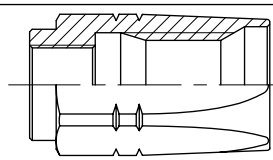
2000-02 ОБЖИМНАЯ ВТУЛКА R2 Рукав со снятием оболочки
