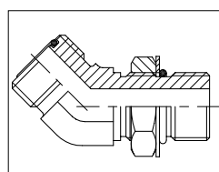
7733 РЕГУЛИРУЕМЫЙ УГЛОВОЙ ФИТИНГ 45°, НАРУЖНАЯ РЕЗЬБА UNF, С СОЕДИНЕНИЕМ SAE O
