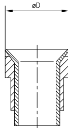
Наружный диаметр зажимной втулки
