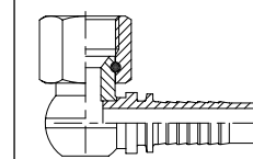
4218~1 Фитинг JIC, компактный, 90°, унифицированная внутренняя резьба, коническое уплотнение 74° Гайка с упорной проволокой
