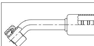
5705 UN 45° FS с уплотнительным кольцом Для рукава AC 1445
