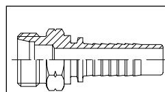
4220 Фитинг прямой, наружная М-резьба, низкое давление, коническое уплотнение 24° Накидная гайка
