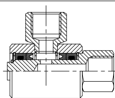
5592 ПОВОРОТНЫЕ МУФТЫ ВЫСОКОГО ДАВЛЕНИЯ, 90°
