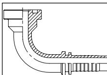
4244 Фитинг 90°, фланцевый, SAE J518 Код 61
